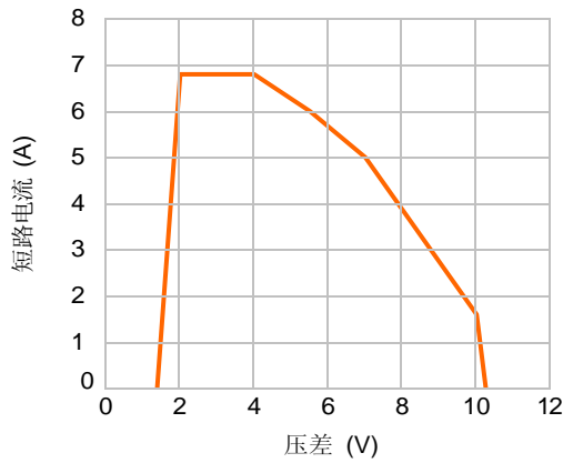
短路电流 vs. 压差
