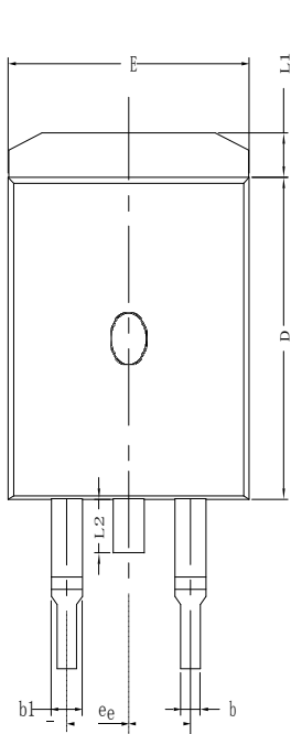
TO-263-2L
