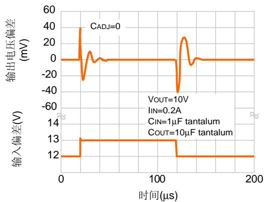
线性瞬态响应
